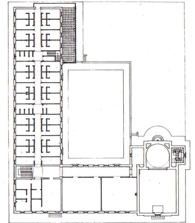
Planta primera
